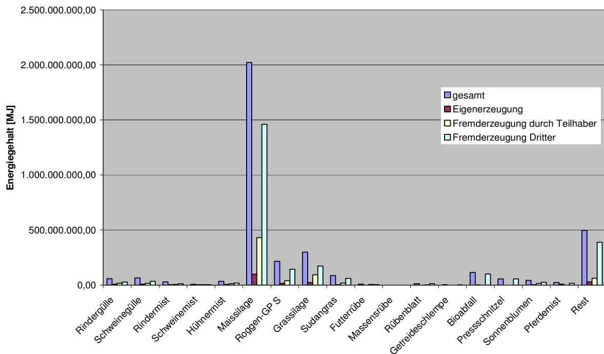
Abbildung 68: Aufteilung nach Energiegehalt (Sample 198 Anlagen)
