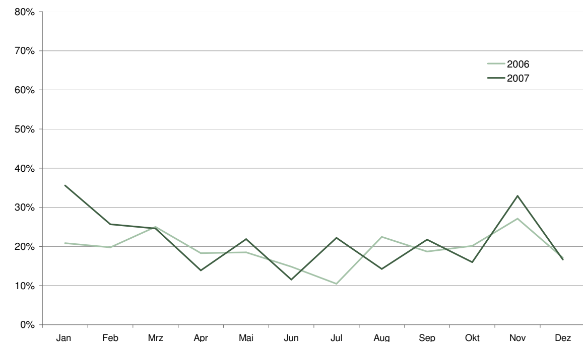
Abbildung 31: Windkraft: monatliche Einspeisemengen (in %) von Windkraftanlagen in den Jahren 2006 und 2007
