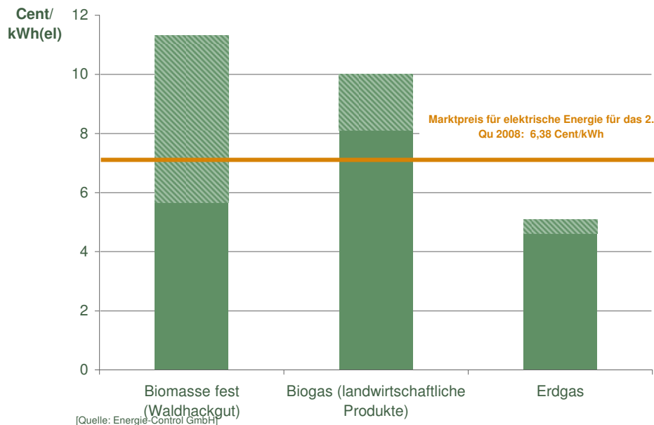
Abbildung 73: Brennstoffkosten (Richtwerte) pro kWh Stromerzeugung für Biomasse (Waldhackgut), Biogas (aus Mais) und Erdgas
