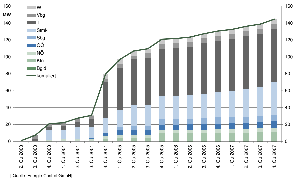
Abbildung 19: Entwicklung anerkannter neuer Kleinwasserkraft-Anlagen vom 2. Quartal 2003 – 4. Quartal 2007
