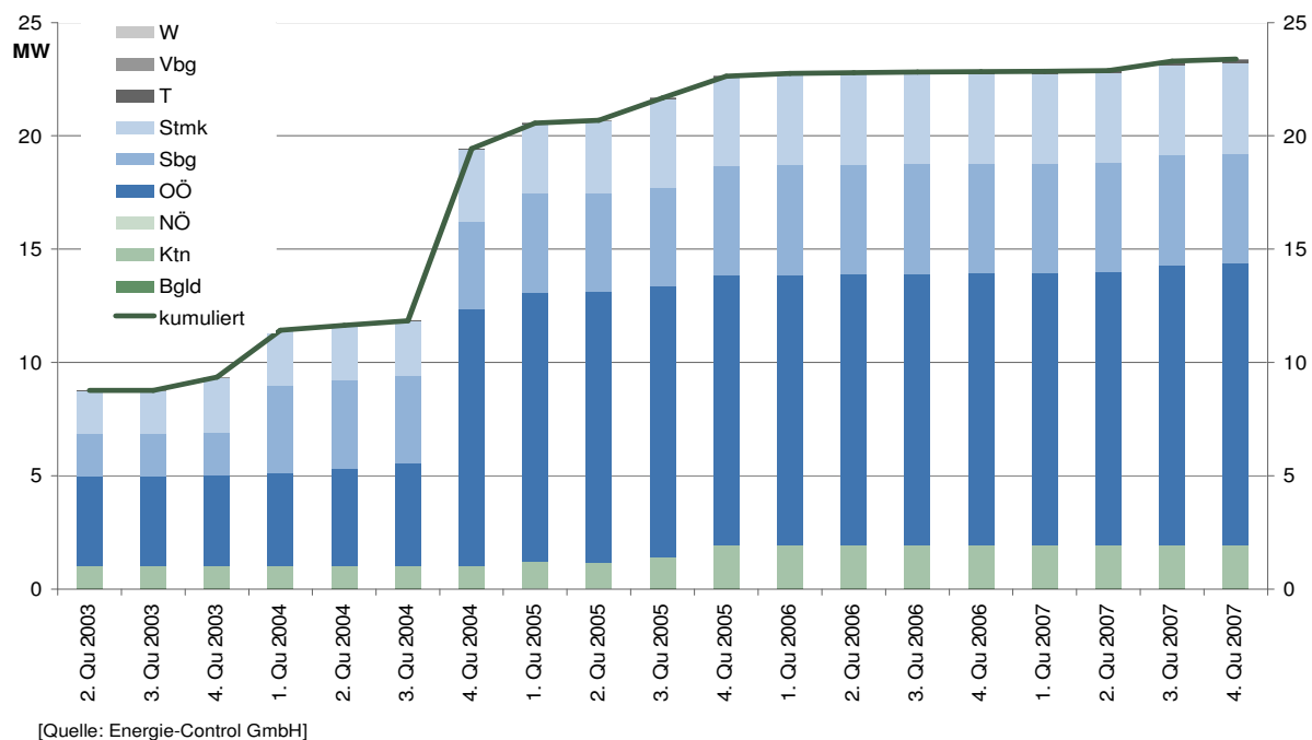
Abbildung 22: Entwicklung anerkannter neuer Kleinwasserkraft-Anlagen aus Revitalisierung (Revitalisierung > 50 %) vom 2. Quartal 2003 - 4. Quartal 2007
