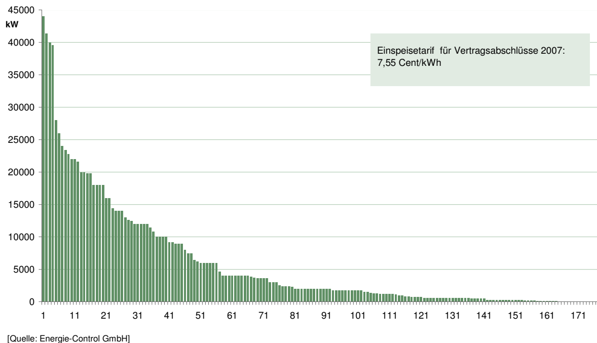
Abbildung 29: Anerkannte Windparks (Summe: 178 Windparks, 1034,1 MW) im Größenvergleich per Ende des 4. Quartal 2007
