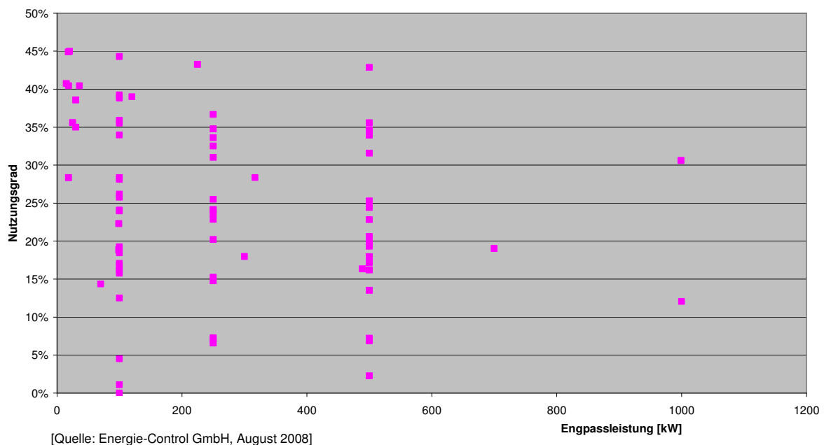
Abbildung 70: Nutzungsgrad Wärme (Sample 79 Anlagen)
