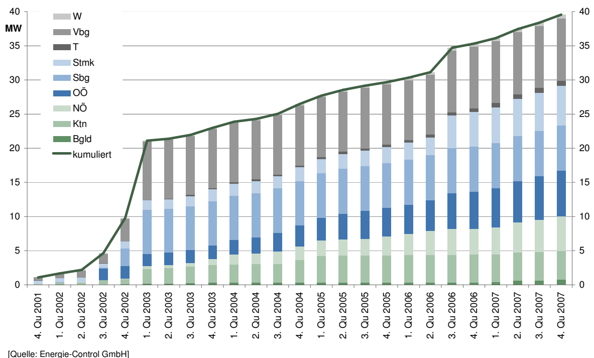
Abbildung 50: Entwicklung anerkannter Photovoltaik-Anlagen vom 4. Quartal 2001 - 4. Quartal 2007
