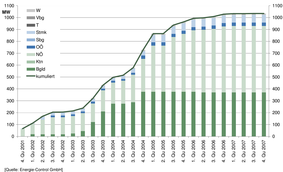
Abbildung 28: Entwicklung anerkannter Windkraft-Anlagen vom 4. Quartal 2001 - 4. Quartal 2007
