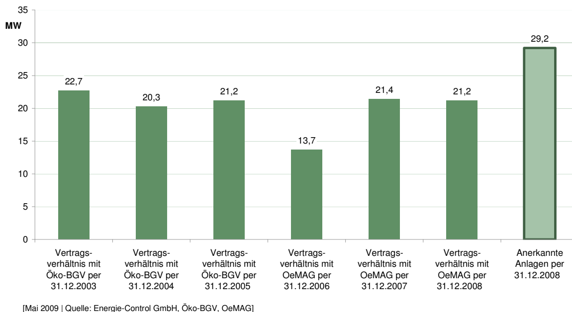
Abbildung 49: Entwicklung der Deponie- und Klärgasanlagen 2003 2008 (gefördert und in Betrieb vs anerkannt)
