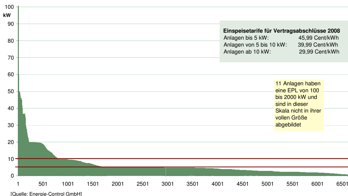
Abbildung 54: Anerkannte Photovoltaik-Anlagen (Summe: 6632 Anlagen, 48,5 MW) im Größenvergleich per Ende des 4. Quartal 2008
