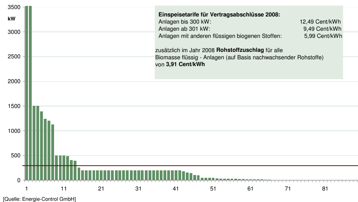
Abbildung 45: Anerkannte Biomasse flüssig-Anlagen (Summe: 90 Anlagen, 26,2 MW) im Größenvergleich per Ende des 4. Quartal 2008
