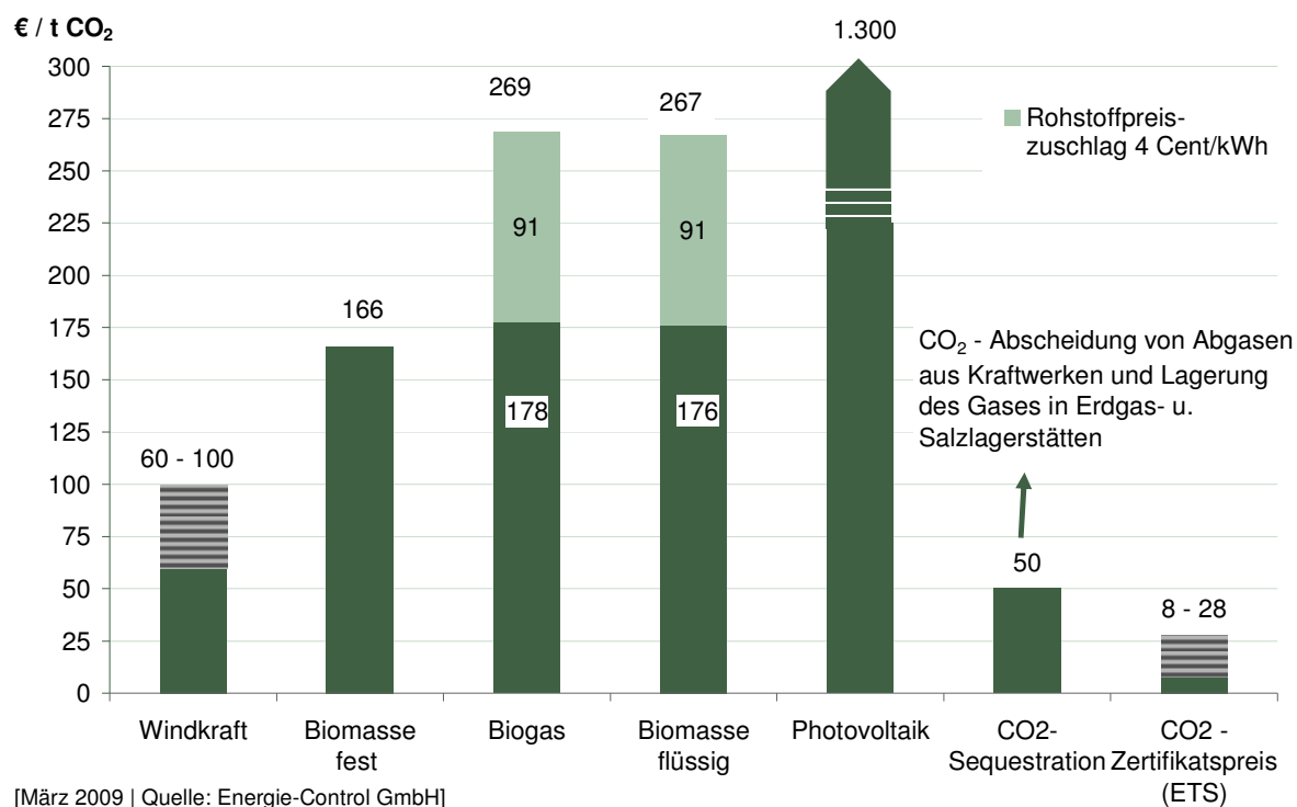
Abbildung 61: CO 2 -Minderungskosten verschiedener Ökostrom-Technologien
