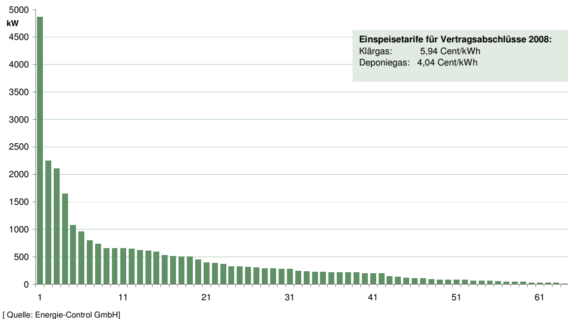
Abbildung 48: Anerkannte Deponie- und Klärgas-Anlagen (Summe: 64 Anlagen, 29,2 MW) im Größenvergleich per Ende des 4. Quartal 2008
