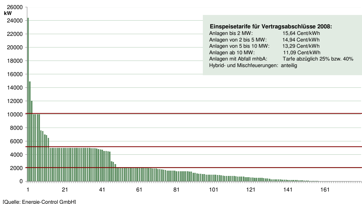
Abbildung 33: Anerkannte Biomasse fest - Anlagen (inkl Abfall mhbA), (Summe 181 Anlagen, 408 MW) im Größenvergleich per Ende des 4. Quartal 2008
