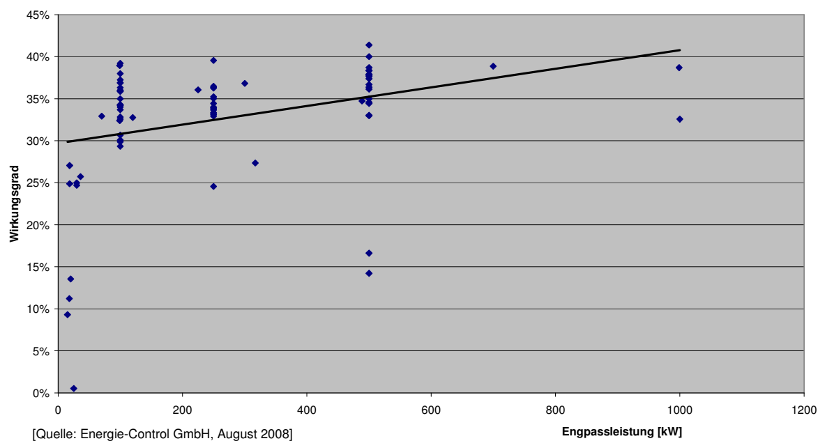
Abbildung 41: Wirkungsgrad Strom (Sample 79 Anlagen)
