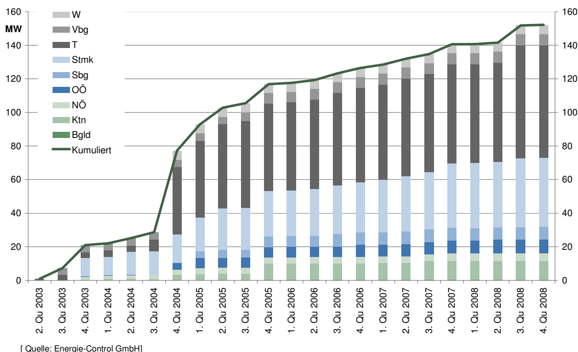
Abbildung 19: Entwicklung anerkannter neuer Kleinwasserkraft-Anlagen vom 2. Quartal 2003 – 4. Quartal 2008
