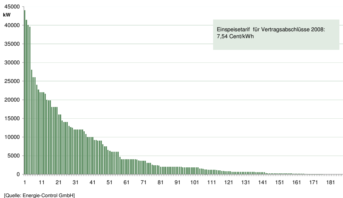
Abbildung 29: Anerkannte Windparks (Summe: 190 Windparks, 1047,8 MW) im Größenvergleich per Ende des 4. Quartal 2008
