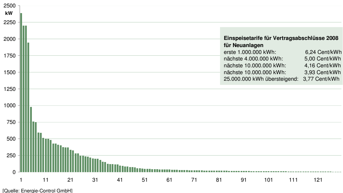
Abbildung 23: Anerkannte neue Kleinwasserkraft-Anlagen aus Revitalisierung, Revitalisierung > 50 %, (Summe: 130 Anlagen, 23,5 MW) im Größenvergleich per Ende des 4. Quartal 2008
