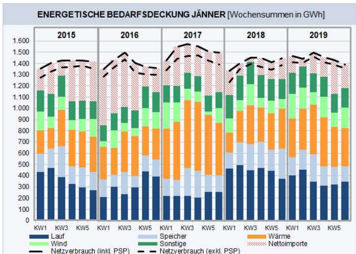
Abbildung 22: Jännervergleich der energetischen Bedarfsdeckung (Regelzone)
