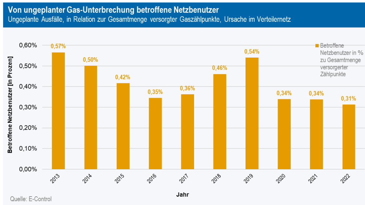
Abbildung 4: Entwicklung von ungeplanter Gas-Unterbrechung betroffene Netzbenutzer mit Ursache im Verteilernetz 2013 bis 2022 [in Prozent]
