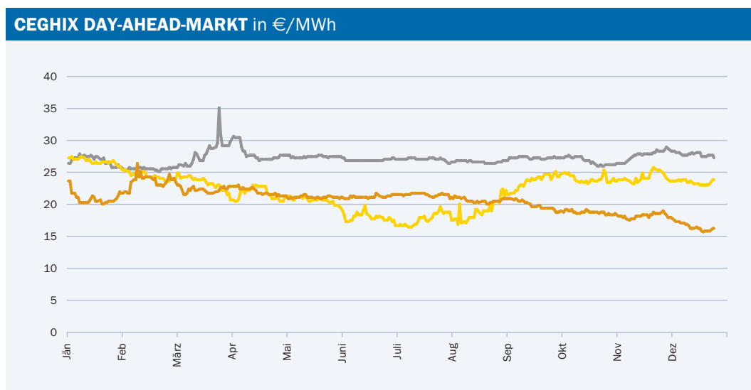
Abbildung 20 CEGHIX Day-ahead-Markt
