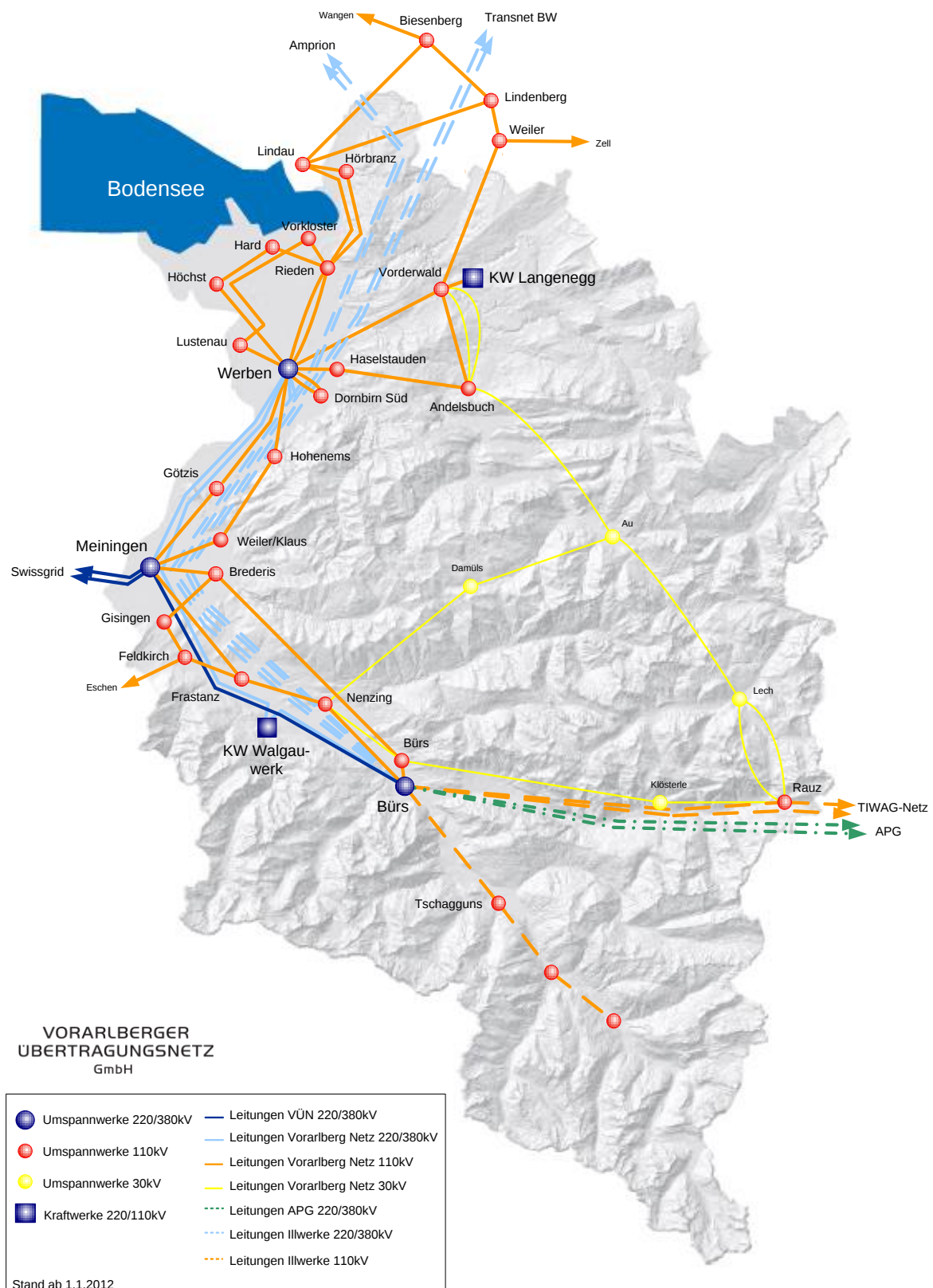
Abbildung 1 Übertragungsnetz in Vorarlberg (inkl. Leitungen von APG, Illwerke und Vorarlberg Netz)
