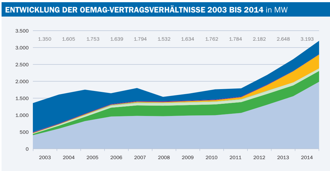
Abbildung 6 Entwicklung der installierten Leistung 8 im Vertragsverhältnis mit der OeMAG 2003 bis 2014
